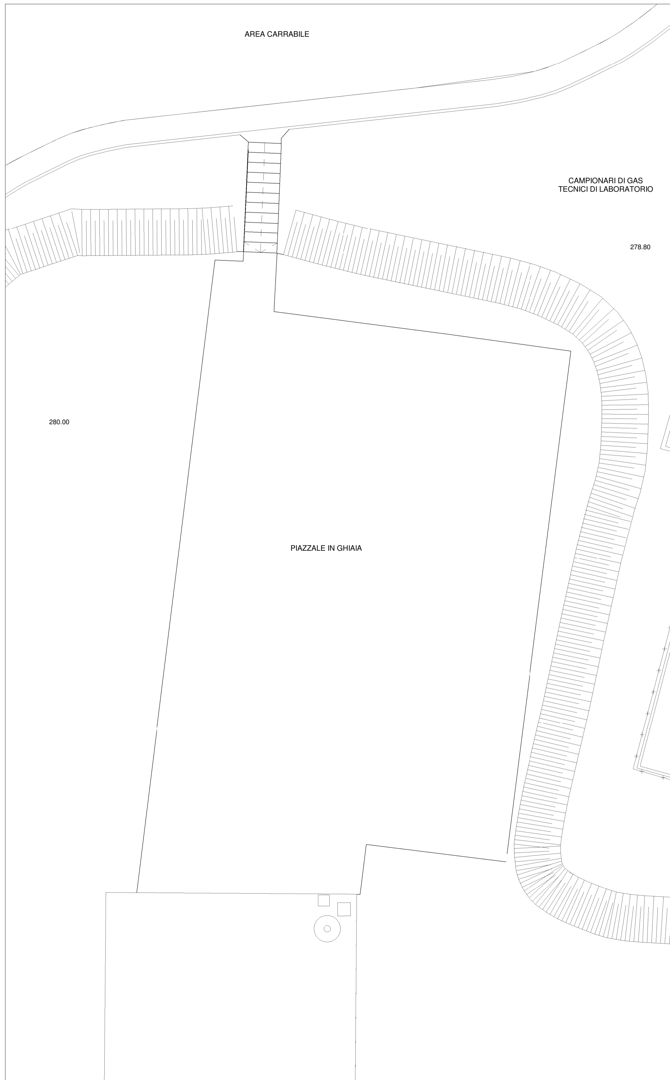
① Planimetria Stato di Fatto 1 : 100
