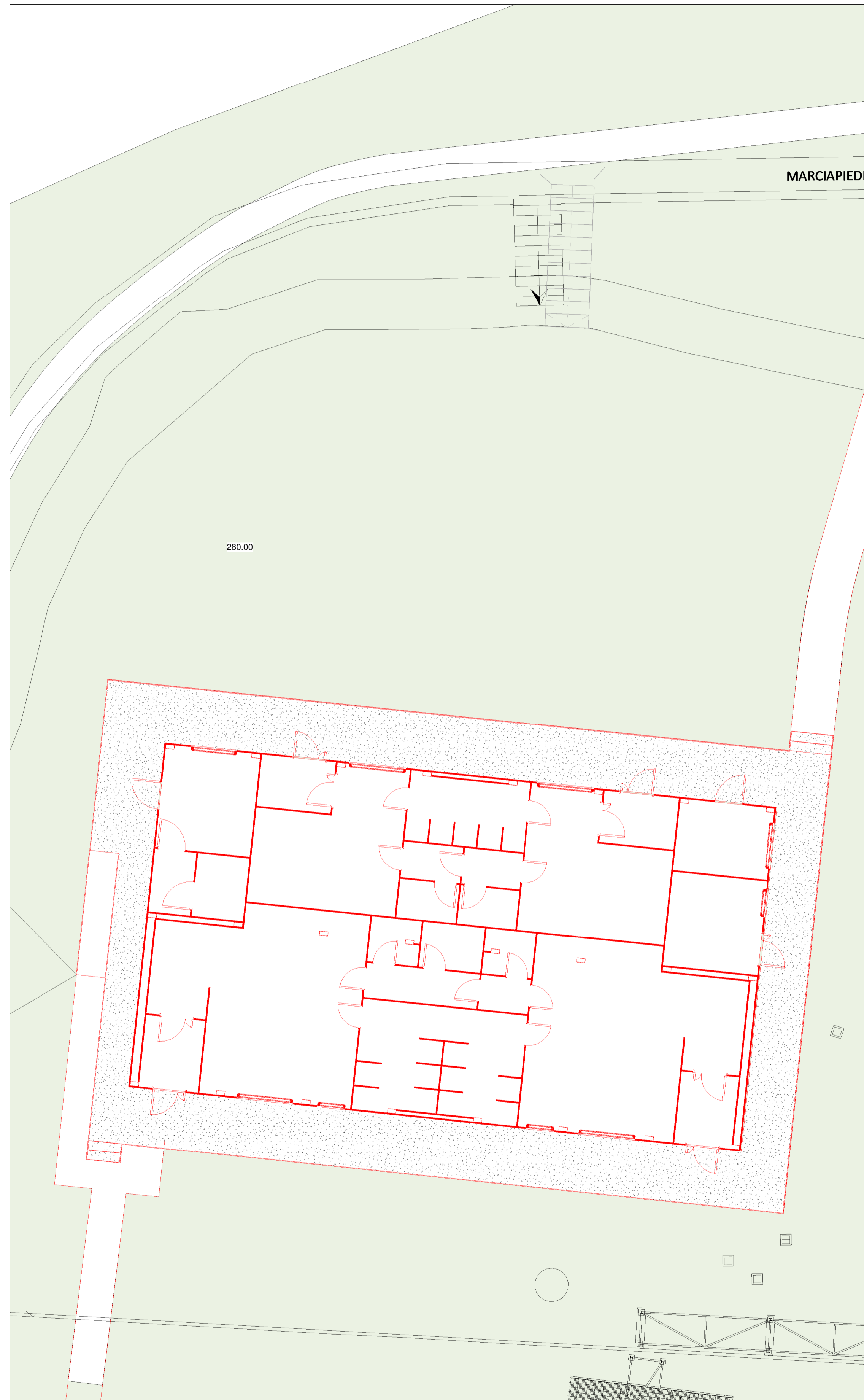
② Planimetria Stato di Progetto 1 : 100
